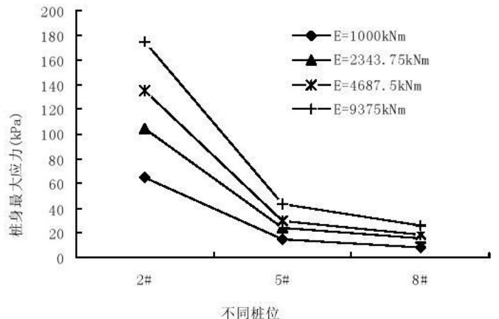
图3 不同桩位桩身最大水平应力衰减情况
