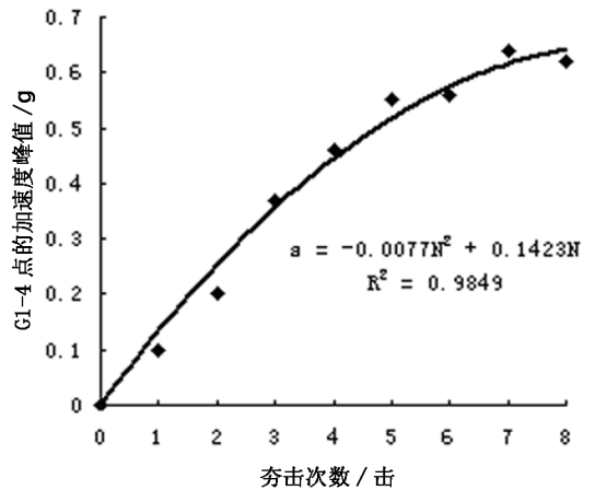
图 4 G1-4 点的加速度峰值与夯击次数的关系
