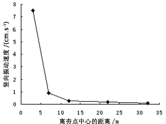
图 9 设置防振沟后地面竖向速度峰值随距离的变化曲线
