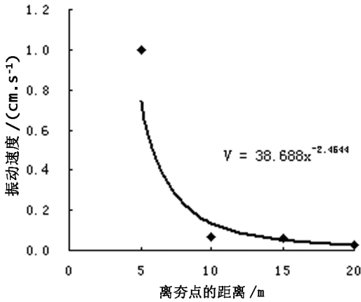
图 6 自由地面竖向速度峰值随距离的变化曲线
