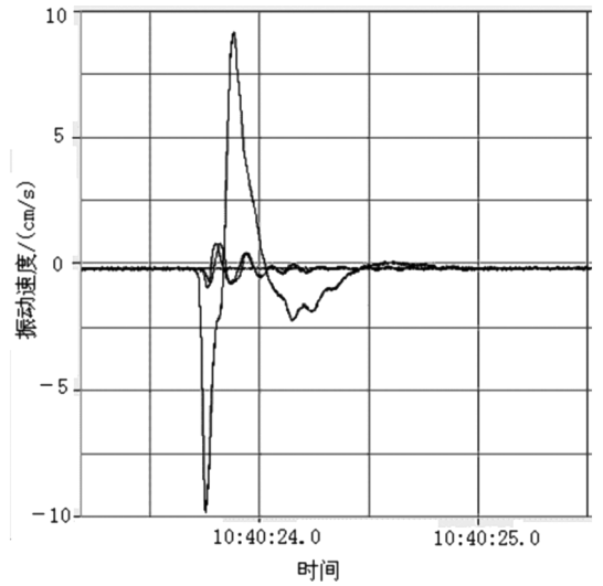
图 7 有防振沟的地面振动速度时程曲线
