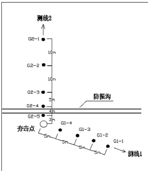
图 3 现场振动测试的测点布置图
