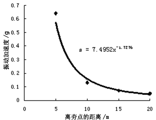
图 5 自由地面竖向加速度峰值随距离的变化曲线
