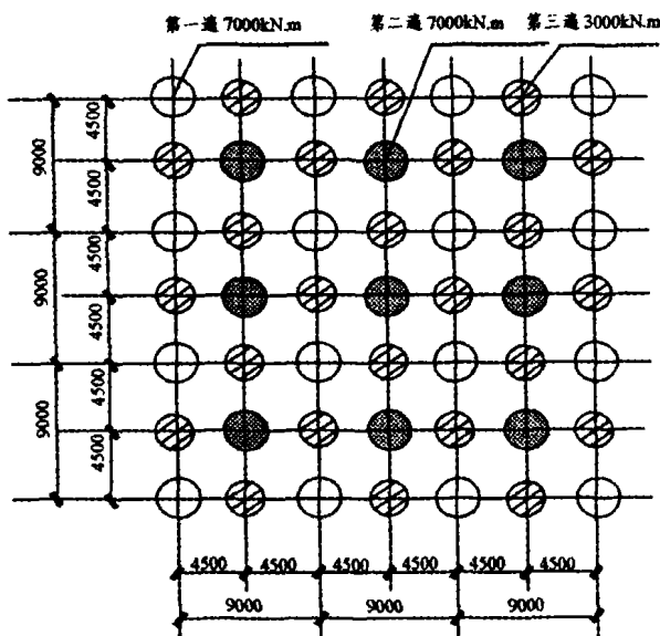
图 1 夯点平面布置图( 7000\text{kN}\cdot\text{m} )
