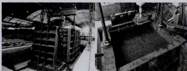
图2 港工结构地基多功能试验模型系统
